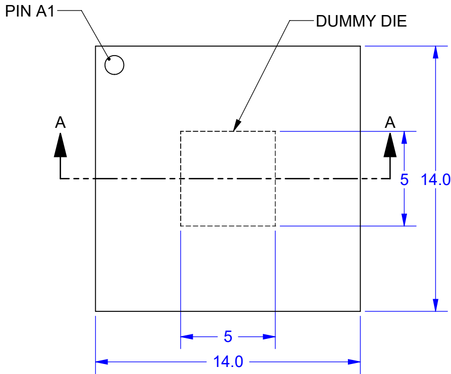
OPTIONAL DUMMY DIE
